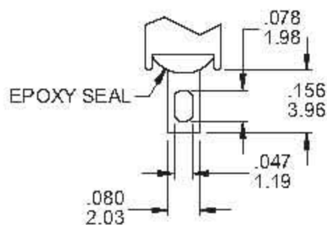
M1 Solder lug
